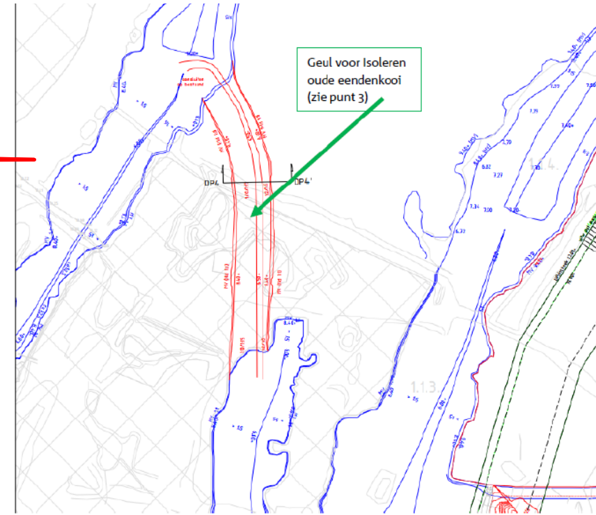
Uitsnede van Tekening nummer 1546 573 0 blad 2
