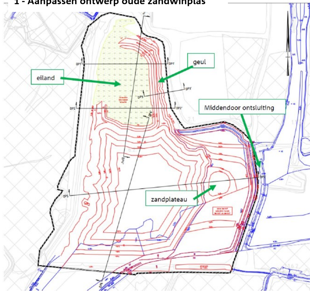
Tekening nummer 1546 586 0 blad 1
